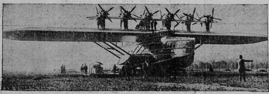
Aquí vemos el gigantesco avión alemán DO-X después de hacer otro vuelo sobre el lago Constanza llevando 169 pasajeros a una velocidad de 105 millas. Se hacen preparativos para un vuelo de este avión a los Estados Unidos próximamente
